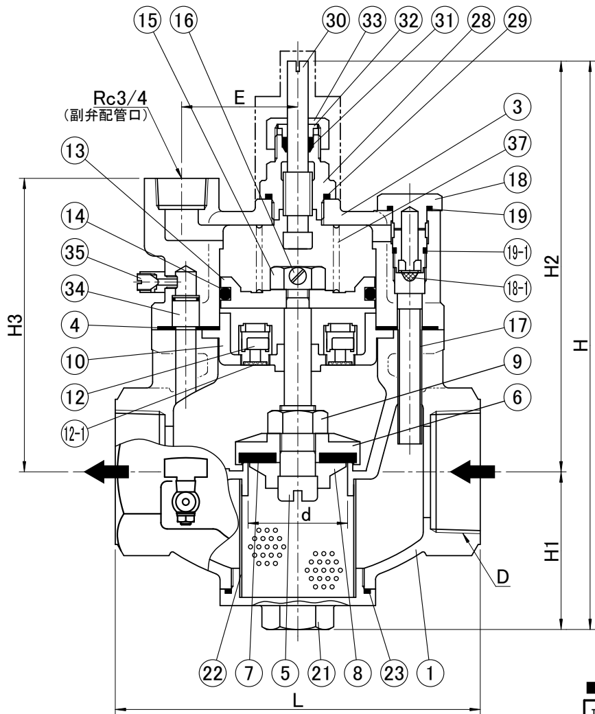
■ 寸法表
