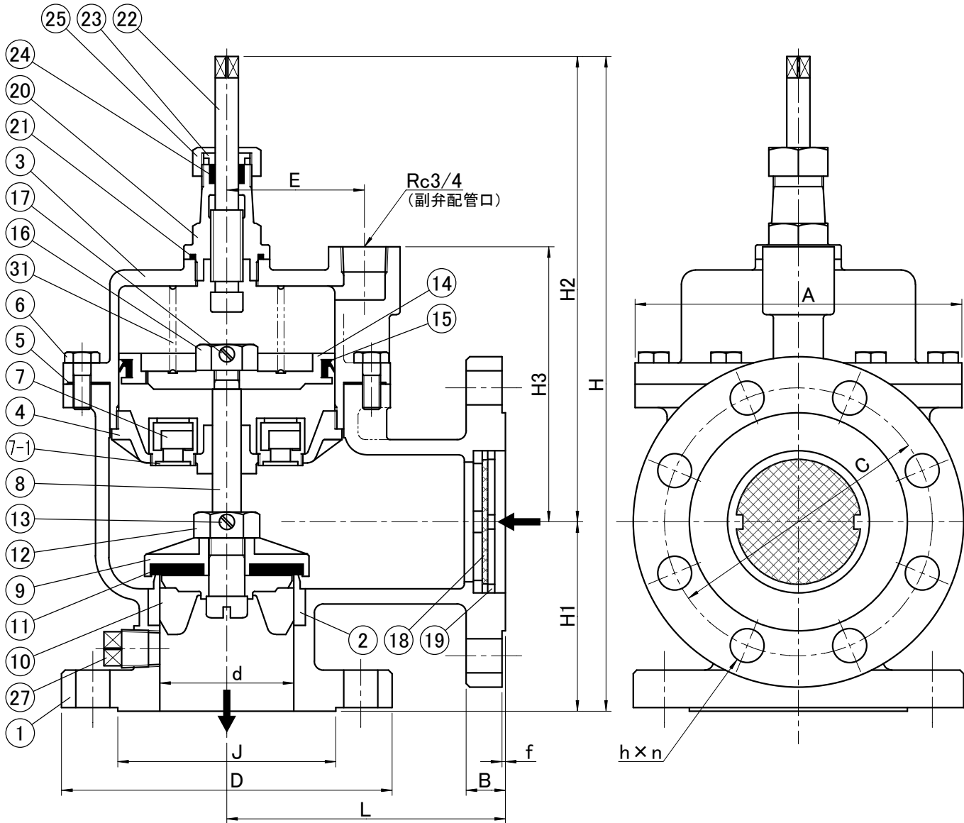
■ 寸法表
